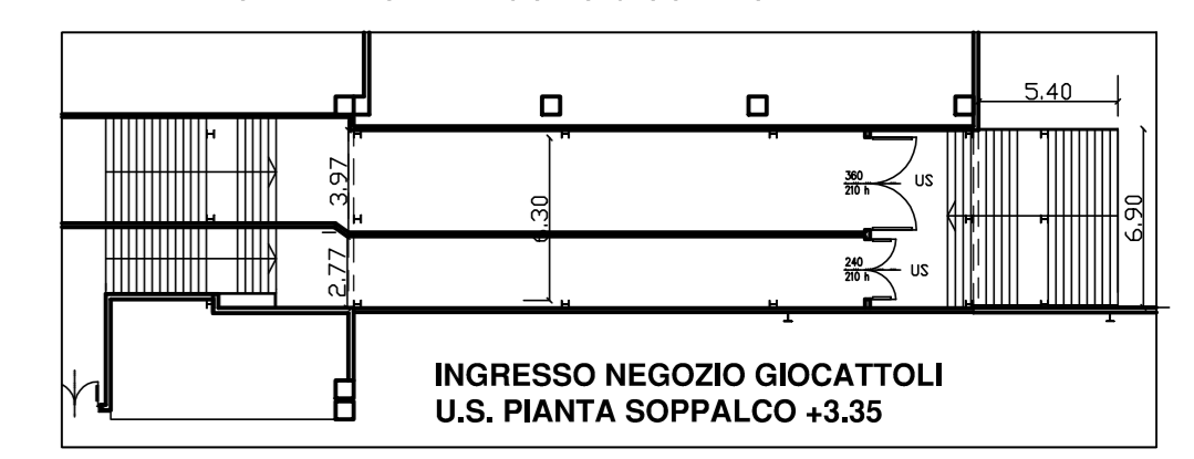
PARTICOLARI USCITA DI SICUREZZA REALIZZATA TRAMITE PIANO INTERMEDIO INTERNO AL NEGOZIO GIOCATTOLI
